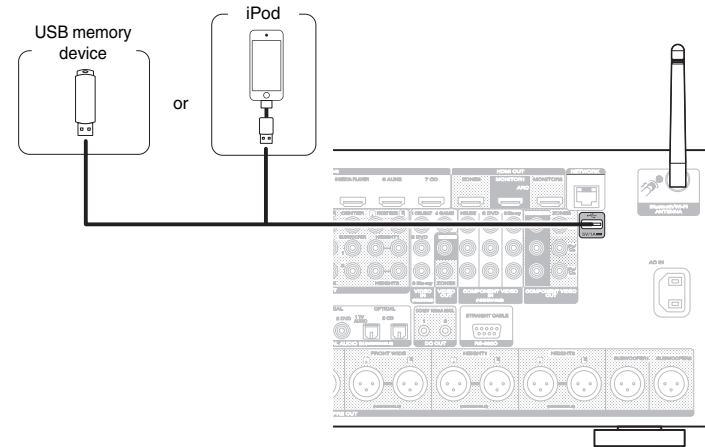
【Rear panel】
